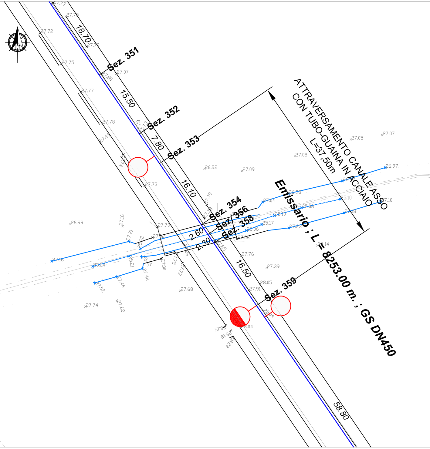
STRALCIO PLANIMETRICO - SCALA 1:500
